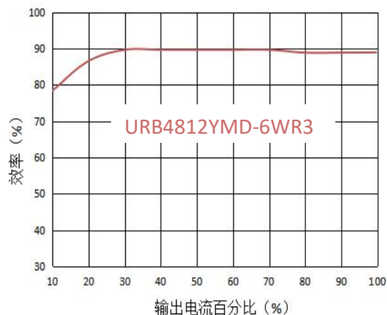
输出效率vs输出负载 (48V输入)
