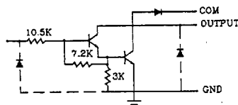
ULN2804
