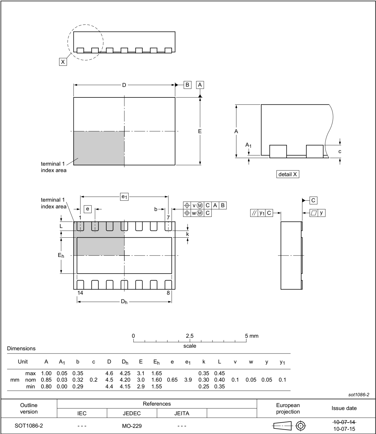
Fig 21. Package outline SOT1086-2 (HVSON14)
