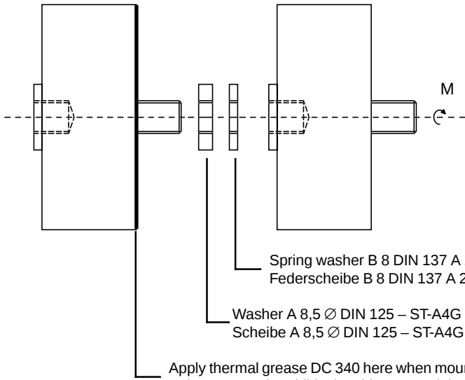
Fig. 7: Mounting of modules Bild 7: Montage der Module
