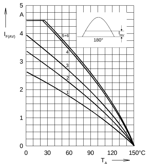
Fig. 4: Load diagramm
