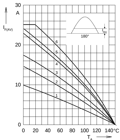
Fig. 4: Load diagramm
