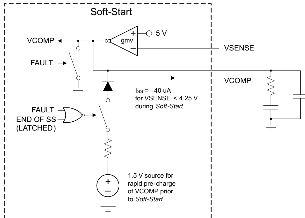
图 23. Soft Start
