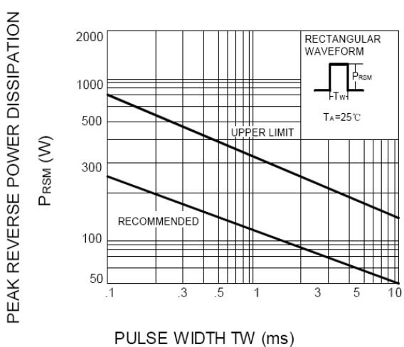
FIG.3 -- P_{RSM} - t_w
