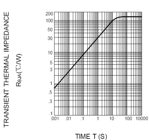
FIG.4 -- R_{\theta JA} - T
