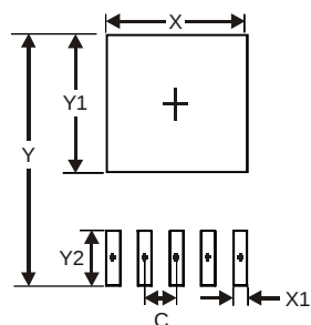
TO263-5
