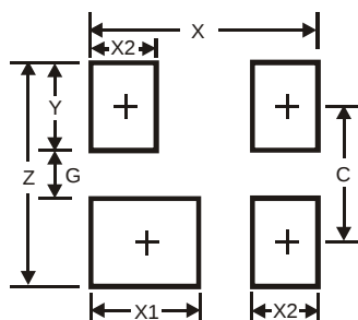
SOT143
