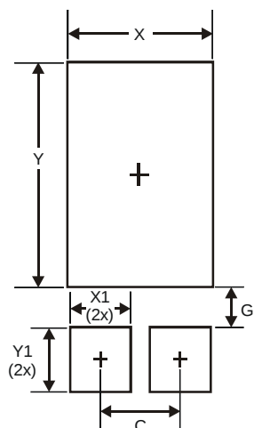
POWERDI®5
