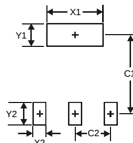
SOT223
