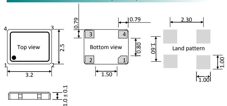
Dimensions (Unit:mm)
