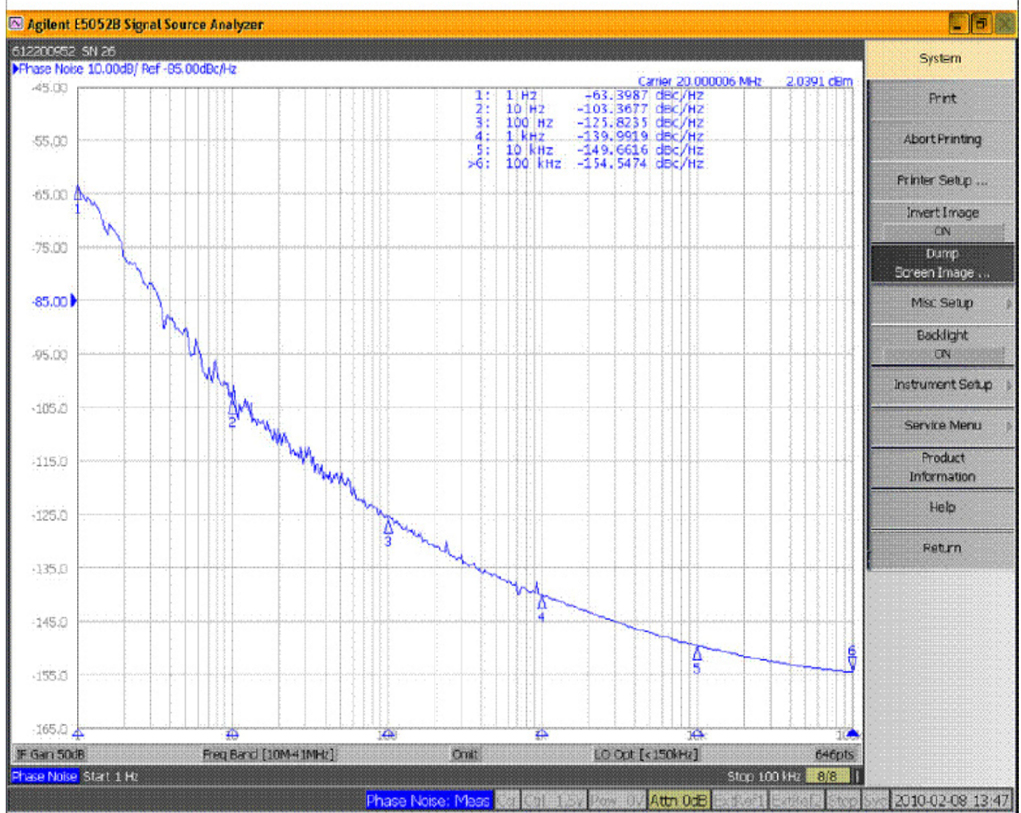
PhaseNoise Plot:
