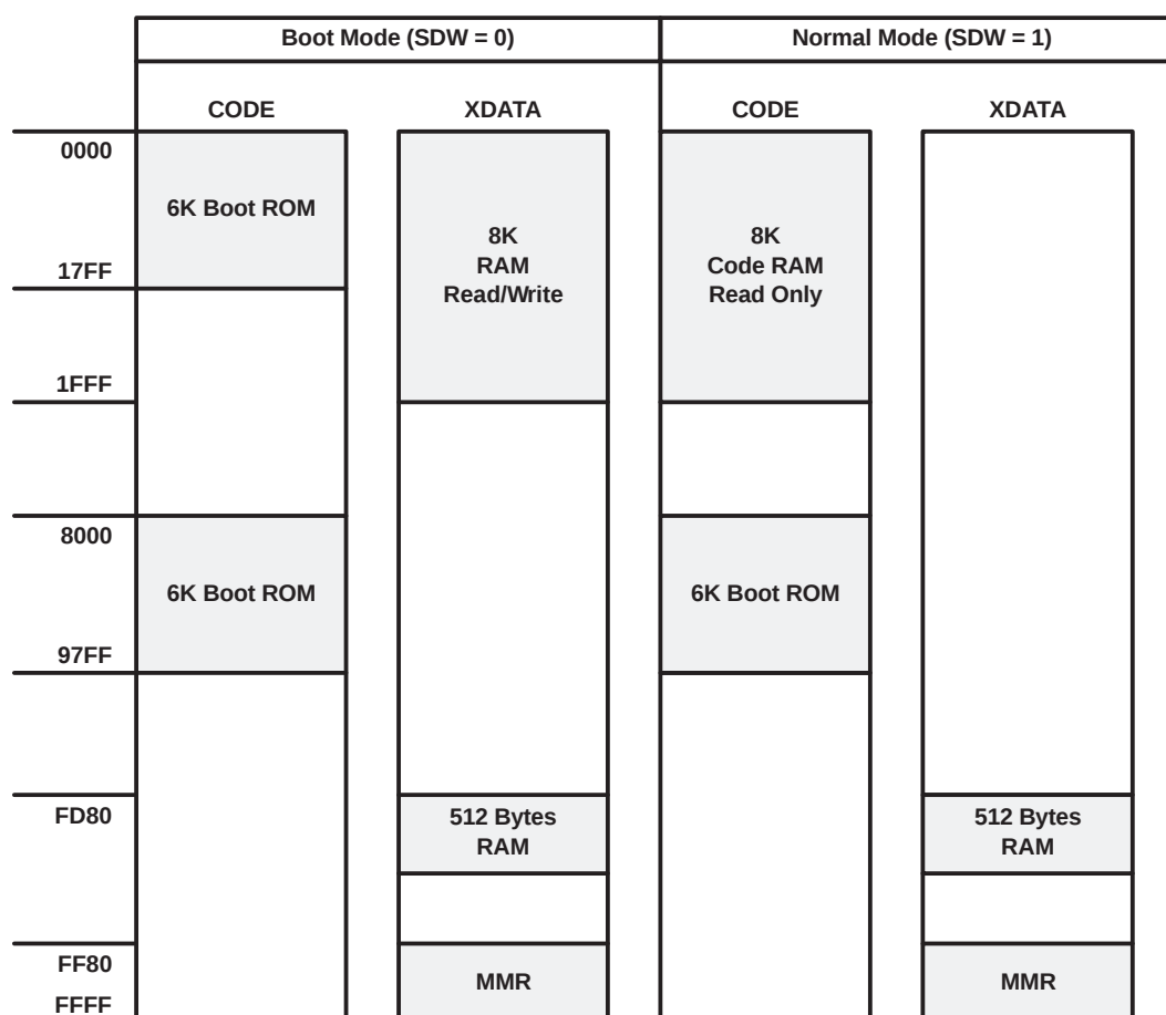
Figure 2-1. MCU Memory Map (TUSB3210)
