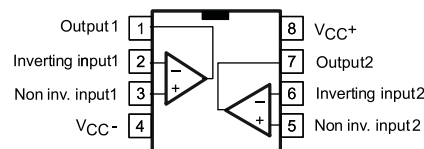
Pin connections TSH82 SO8/TSSOP8
