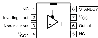
Pin connections TSH81 SO8/TSSOP8
