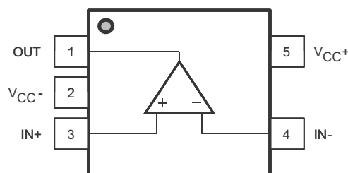
SOT23-5
