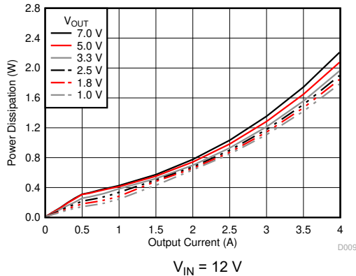
图 6-9. Power Dissipation versus Output Current
