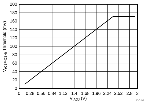
Figure 17. V_{(CSP-CSN)} Threshold vs V_{IADJ}
