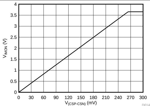
Figure 15. V_{IMON} vs V_{(CSP-CSN)}
