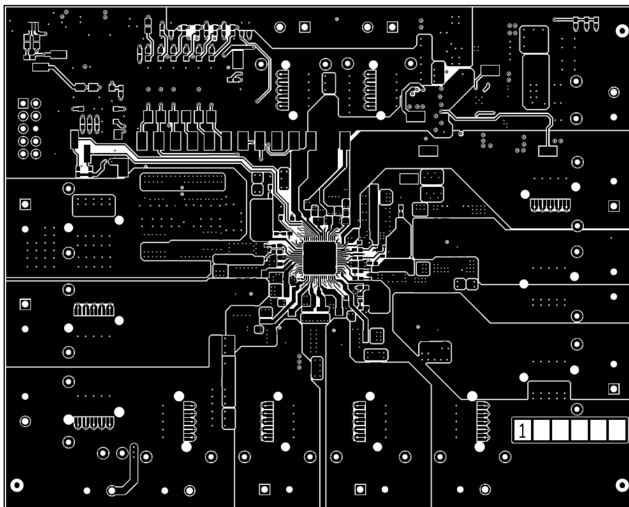
Figure 16. Top Layer
