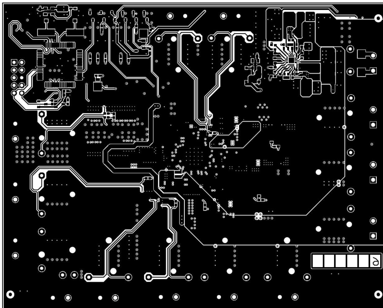
Figure 21. Bottom Layer
