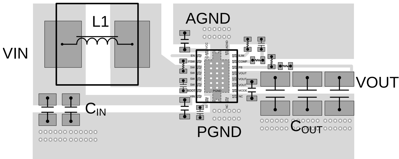
Figure 20. Bottom Layer
