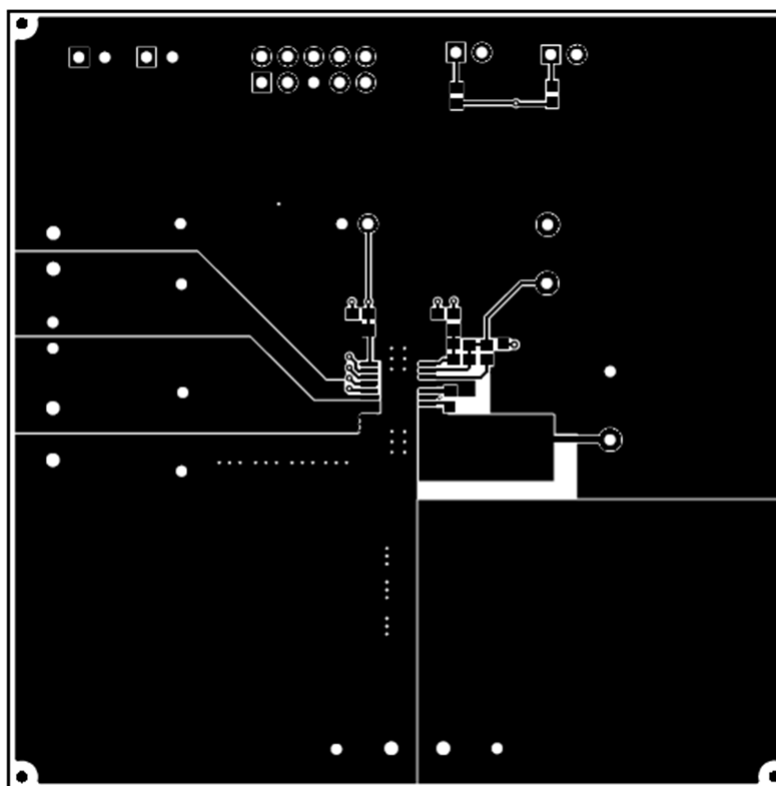
Figure 16. Top Layer
