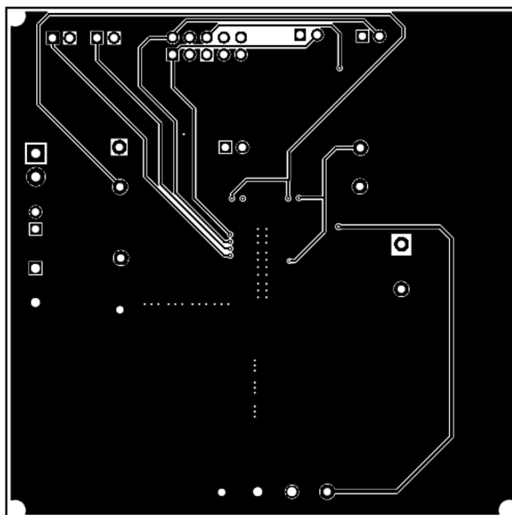
Figure 19. Bottom Layer
