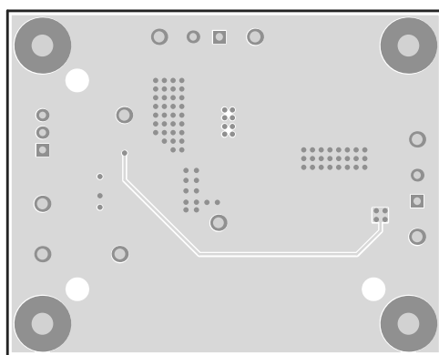
Figure 18. Bottom Layer
