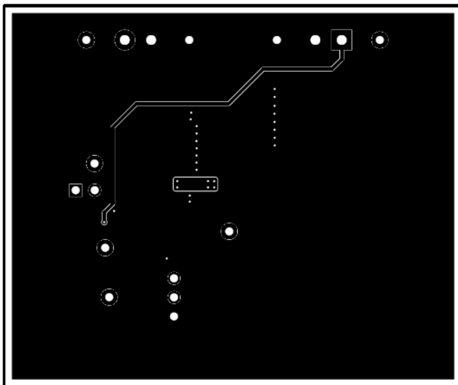
Figure 17. Bottom Layer
