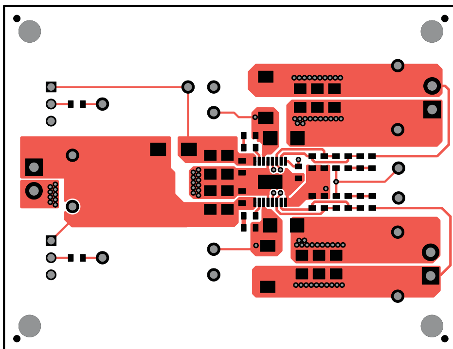
Figure 21. Top Layer
