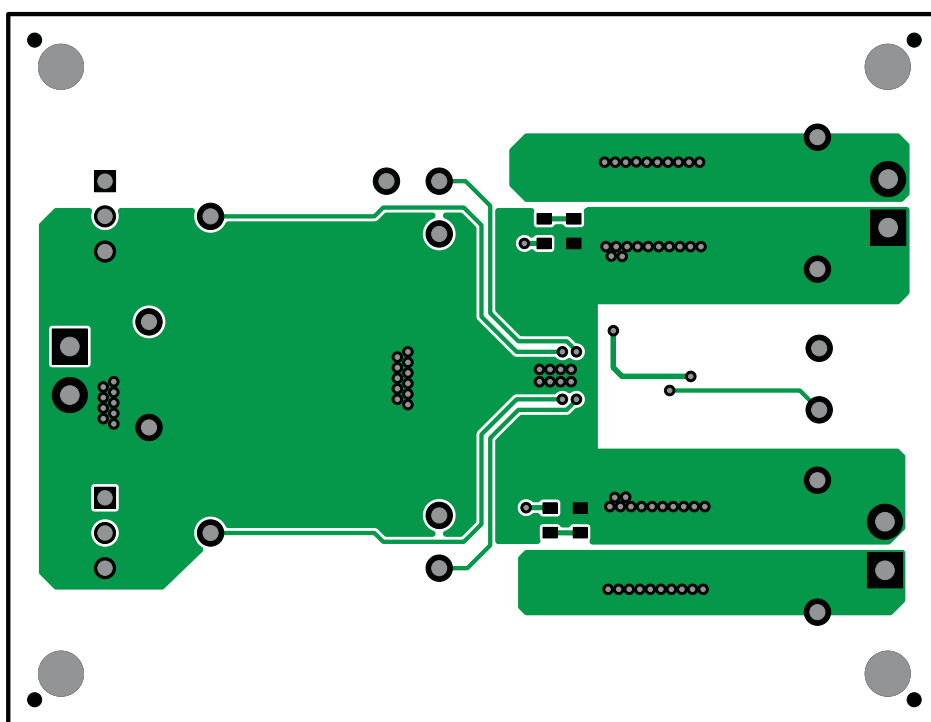
Figure 24. Bottom Layer
