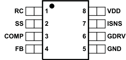
8 PINS SOIC (D) PACKAGE (TOP VIEW)
