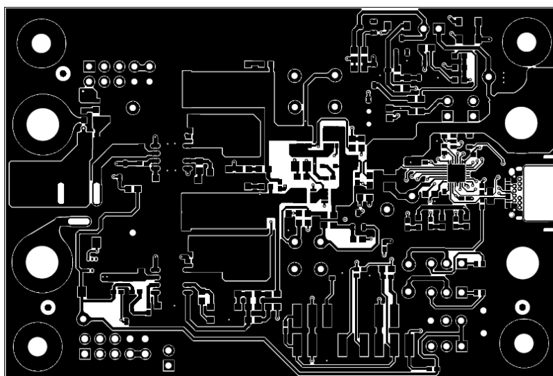
Figure 25. Top Layer
