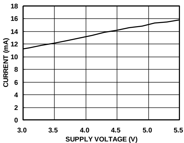
图10. 电源电流与电源电压的关系
