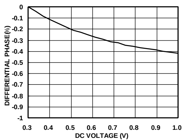
图 14. 微分相位(dP)
