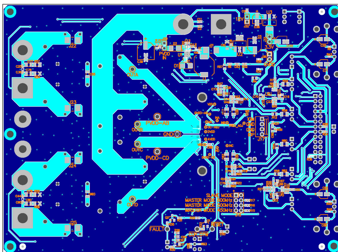
Figure 29. TPA3245 EVM Bottom Layer
