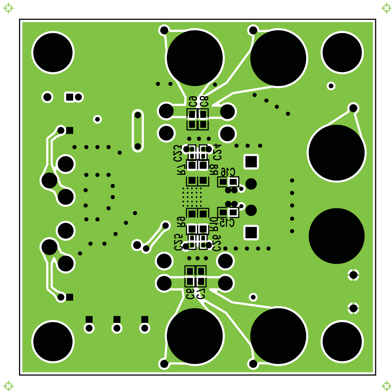
Figure 5. TPA3101D2 Rev.A EVM – Bottom Layer
