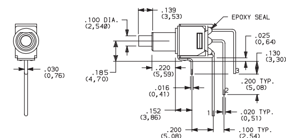
TP12SH9AVBE SPDT
