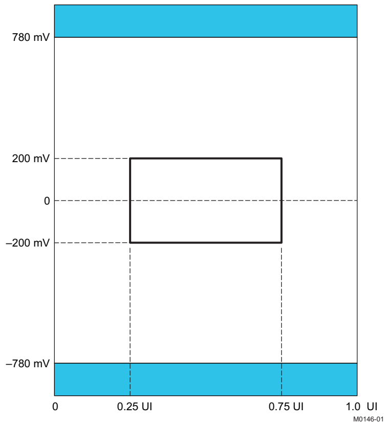
Figure 25. Output-Eye Mask at TTP4
