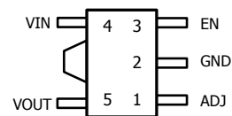
SOT-89-5L
