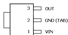
SOT223-3L
