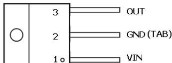
TO220-3L
