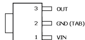
SOT223-3L
