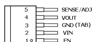
TO263-5L
