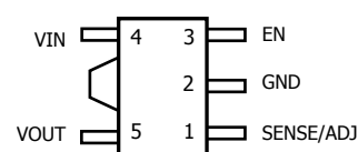
SOT89-5L
