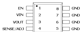
MSOP8 / SOP8
