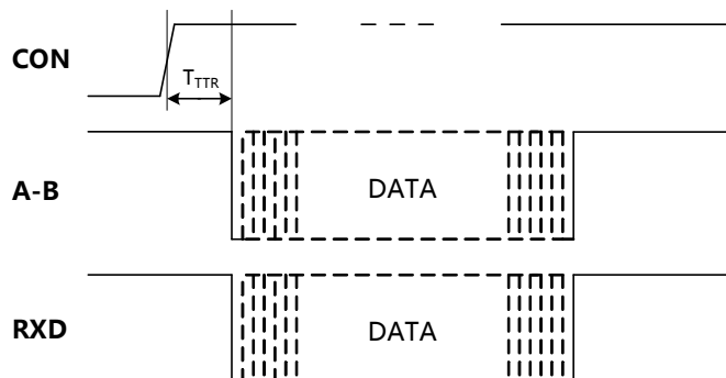
图 2. TDx01D485H-E模块数据接收时序图
