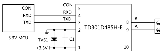
图 4.MCU 3.3V 供电应用电路
