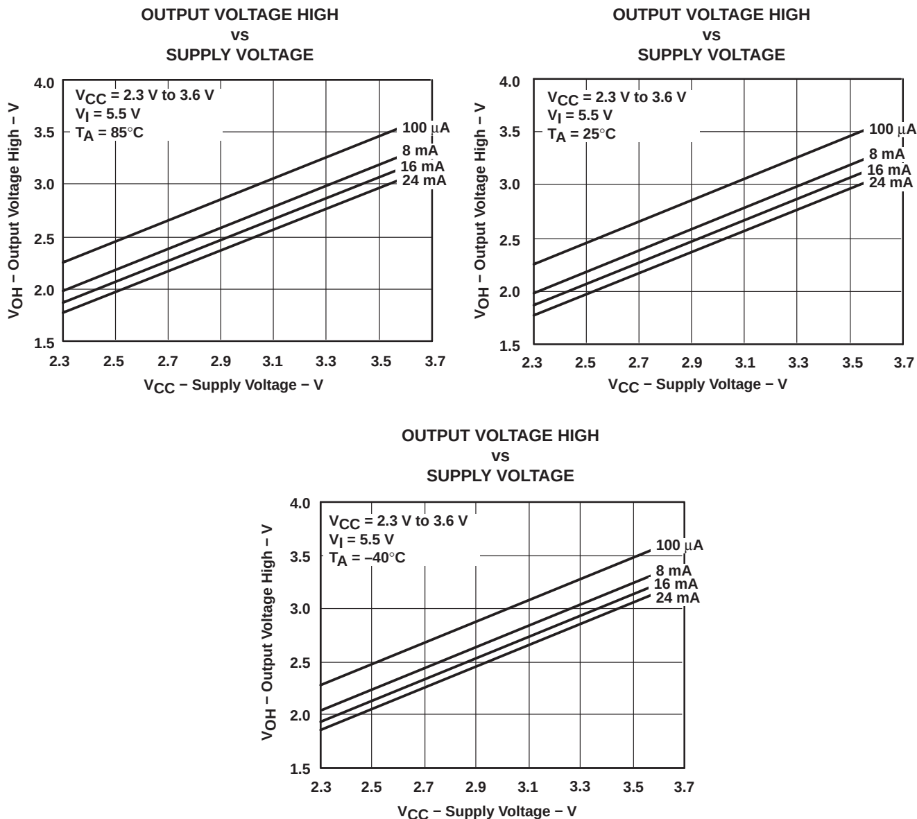
Figure 4. V_{OH} Values
