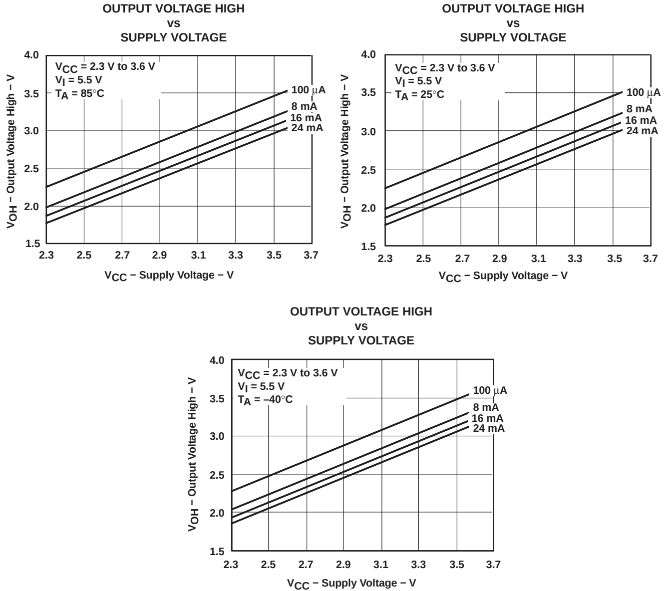
Figure 4. V_{OH} Values
