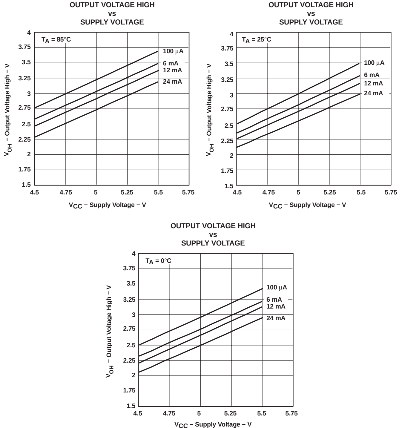
Figure 2. V_{OH} Values
