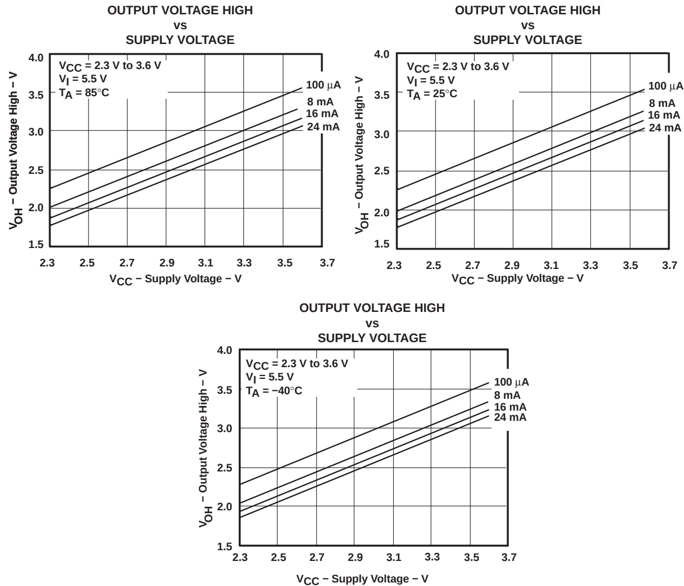
Figure 4. V_{OH} Values
