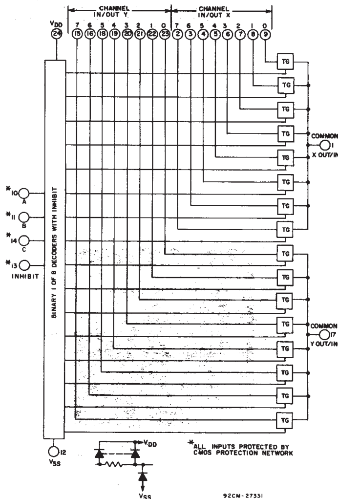
Fig. 17— CD4097 logic diagram.
