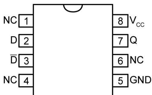
8-Pin SOIC (Z8-1)
