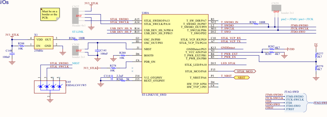
Figure 44. STLINK-V3E -SWD Module
