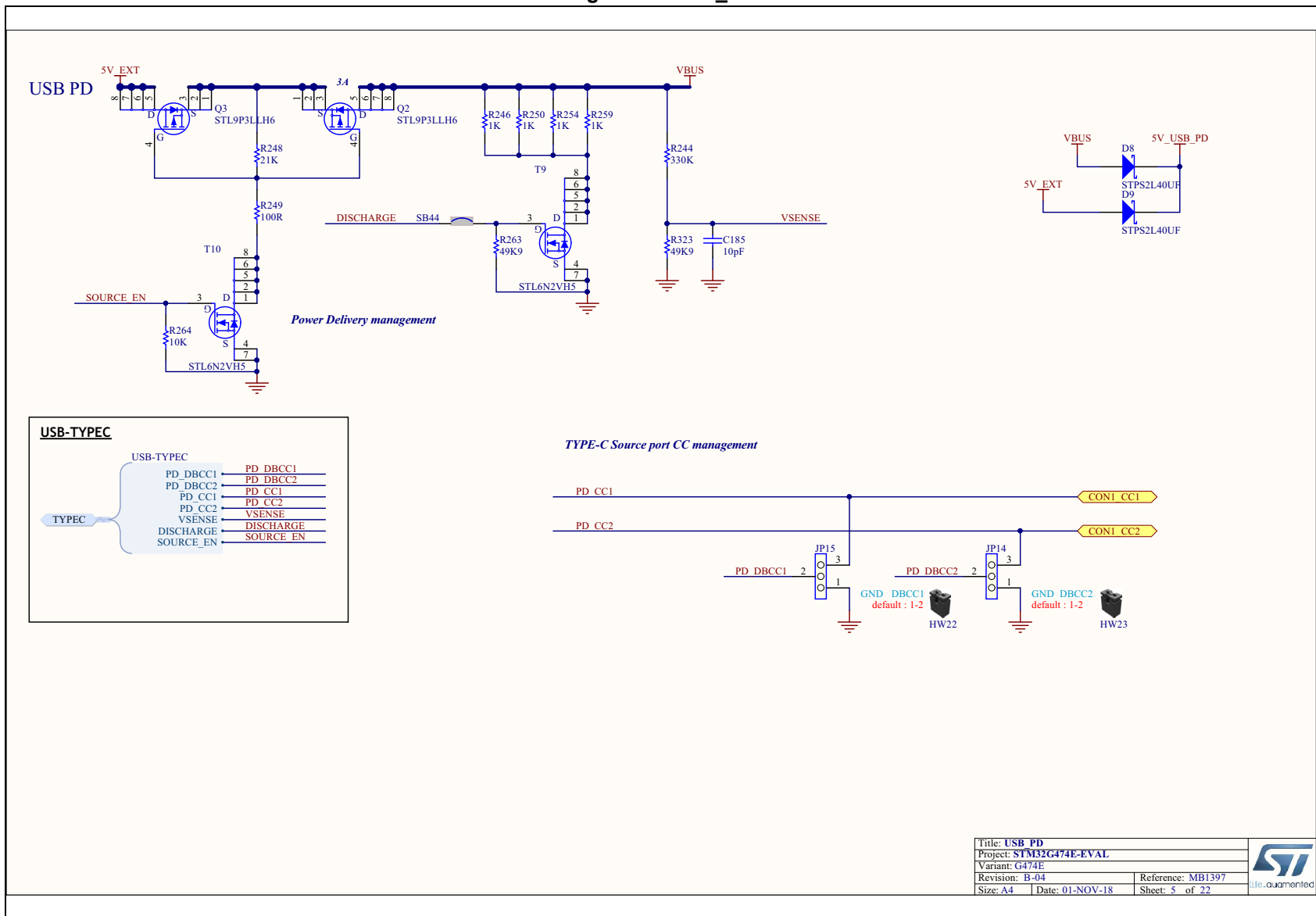
Figure 28. USB_PD
