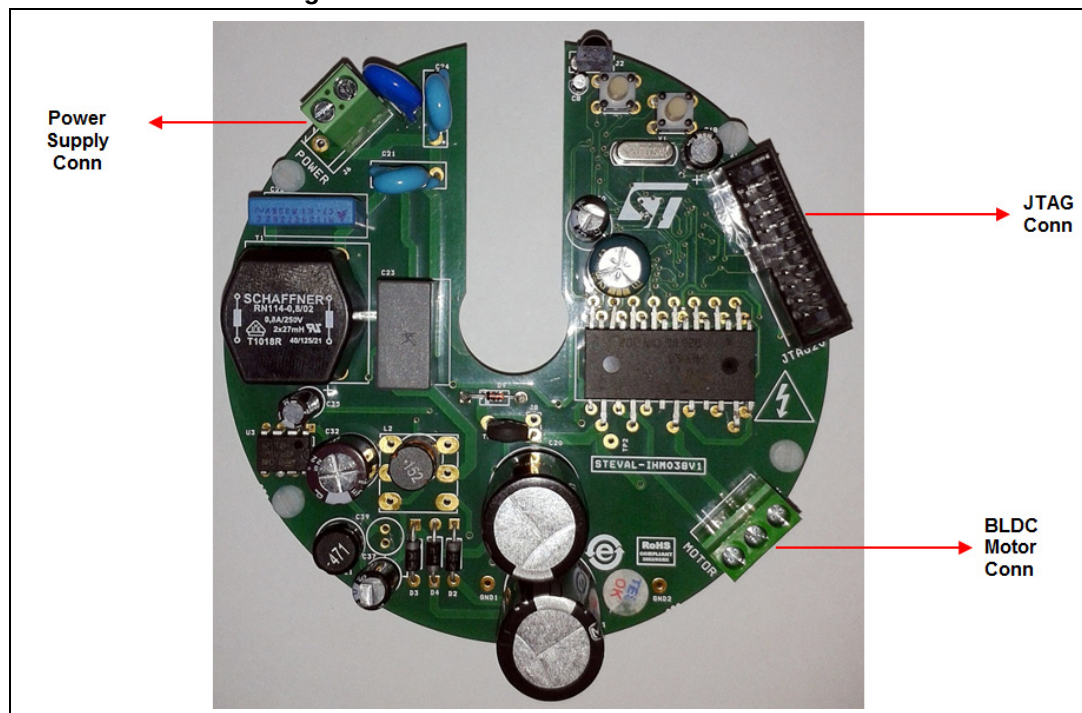
Figure 11. STEVAL-IHM038V1 actual board
