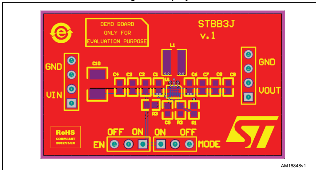
Figure 28. Top layer
