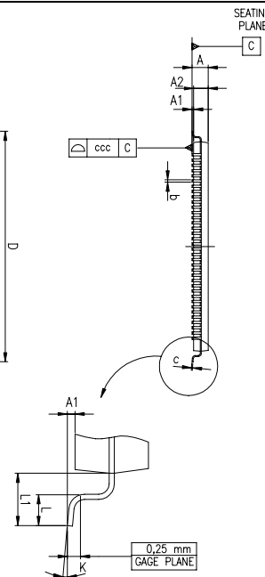
TQFP144 (20x20x1.40mm)
