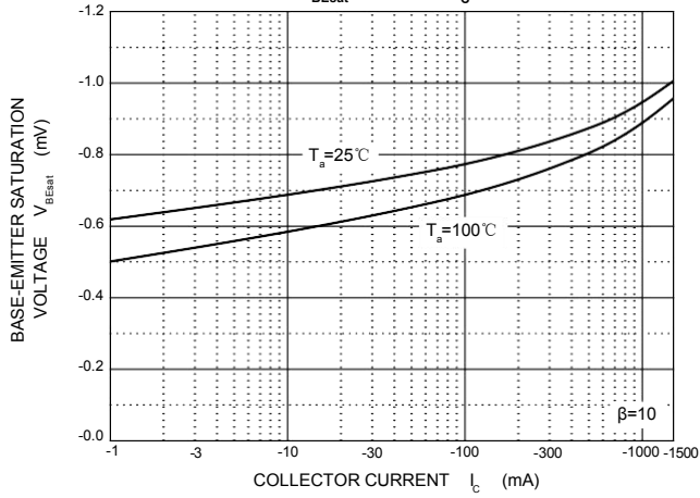
V_{BE} — I_C
