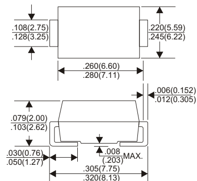
DO-214AB(SMC)
