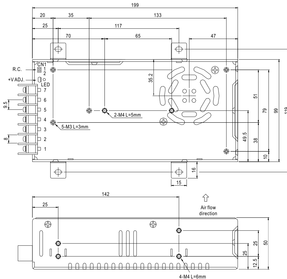
Remote ON/OFF(CN1):JST S2B-XH or equivalent(optional)
