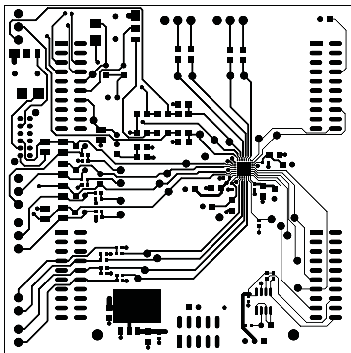
Figure C-2. Top Layer
