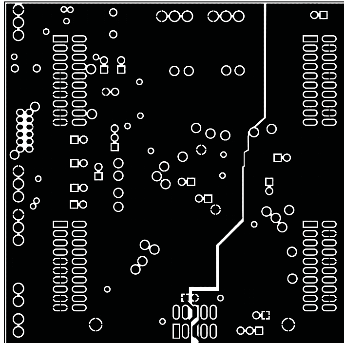
Figure C-3. Layer 3
