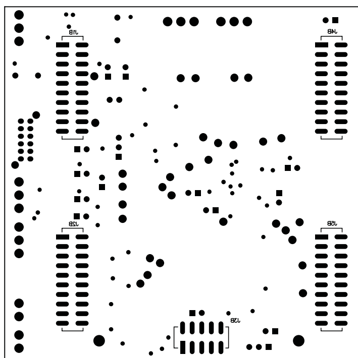
Figure C-6. Bottom Layer
