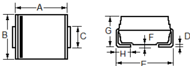
SMB (DO-214AA)
