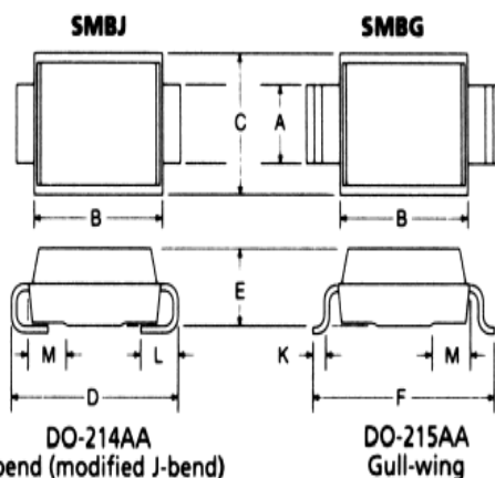
DO-214AA C-bend (modified J-bend)
