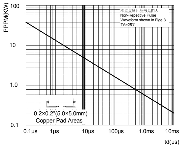
图3: 脉冲波形
