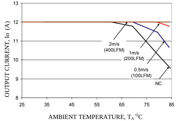
V_o=1.2V
