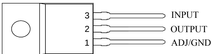
PKG : TO-220F-3L
