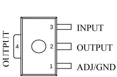
PKG : SOT-89
