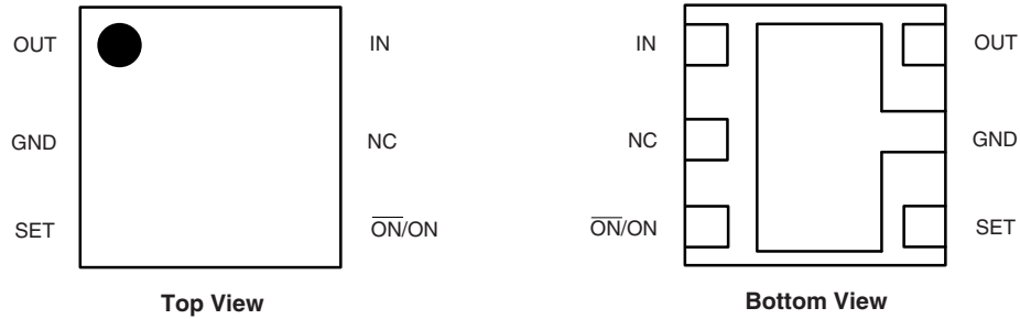
TSC75-6 Package
