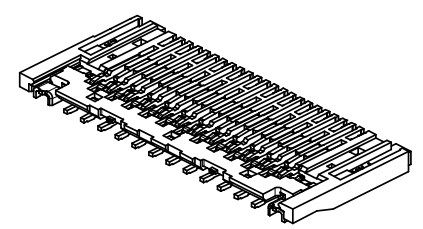
アクチュエータ CLOSE (製品納入状態)
