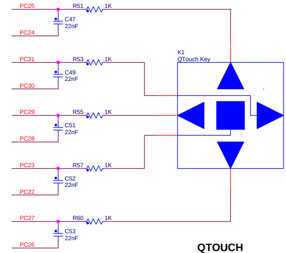
QTOUCH
