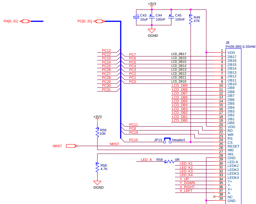
LCD
