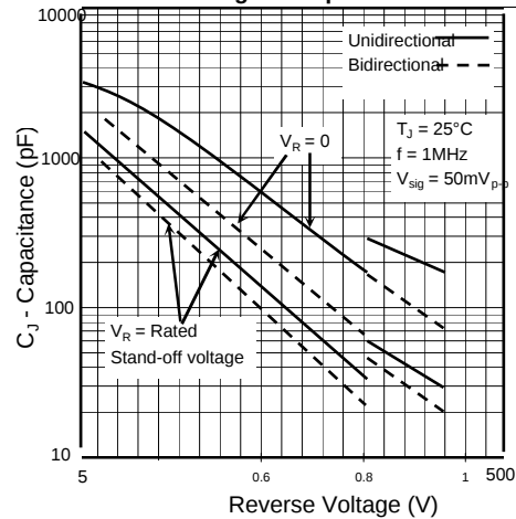
Fig. 6 - Capacitance
